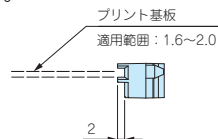
取付穴寸法図 (取付部推奨板厚: 2.0mm)
