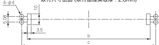
取付穴寸法図 (取付部推奨板厚: 2.0mm)
