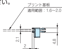
取付穴寸法図 (取付部推奨板厚: 2.0mm)
